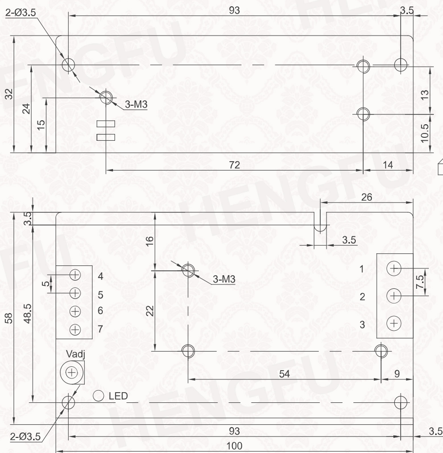
机壳 Frame
